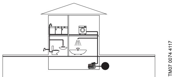
Фиг. 11 Покачване на налягането от водопроводната мрежа
