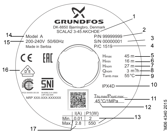
Фиг. 13 Пример за табелка с данни
